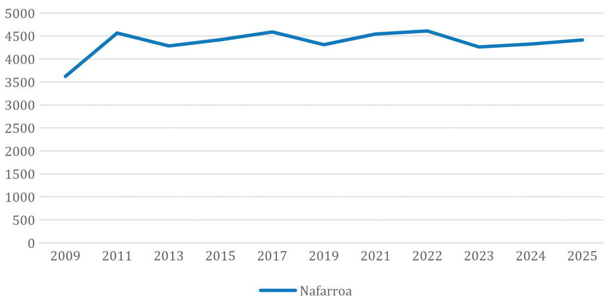
Grafikoa 15: Nafarroako energia kontsumoaren bilakaera (milioi kWh 4 ) (2009-2025)
